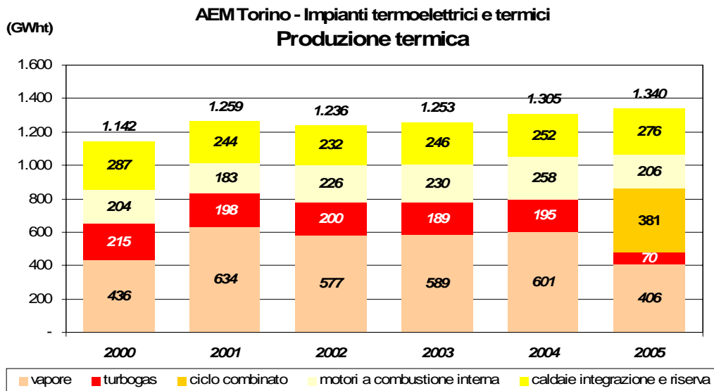
Figura 6 Produzione termica degli impianti di AEM Torino
